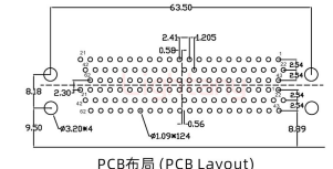
PCB布局 (PCB Layout)
