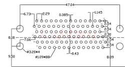
PCB布局 (PCB Layout)
