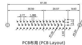
PCB布局 (PCB Layout)
