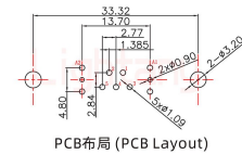
PCB布局 (PCB Layout)
